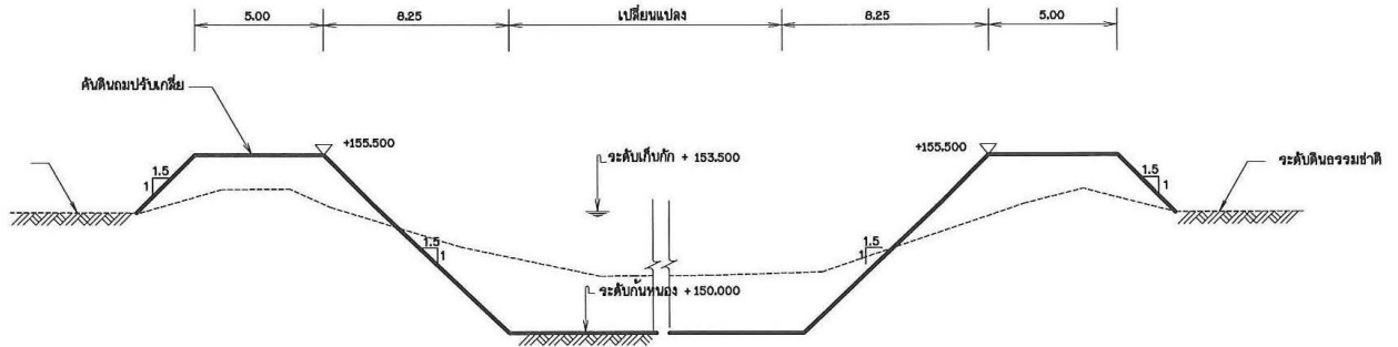
รูปตัดทั่วไป มาตราส่วน 1:100 แนวตั้ง 1:100 แนวนอน 1:200
