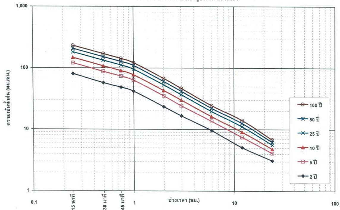
32. IDF Curve สำหรับ อ.อรัญประเทศ จ.สระแก้ว
