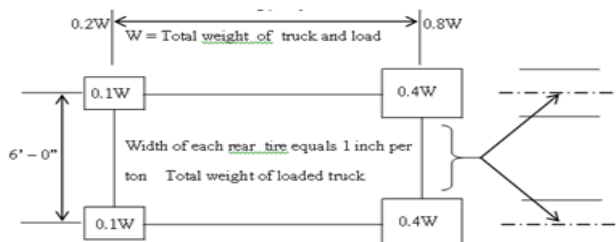
AASHTO Truck Loading
