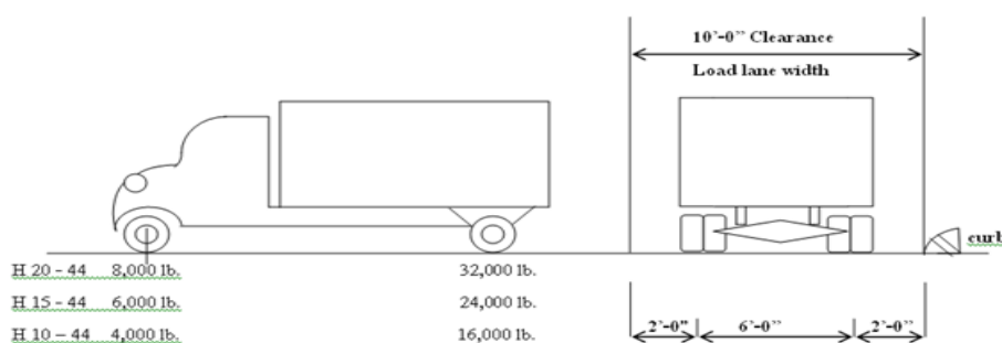
การกระจายของ WHEEL LOAD
