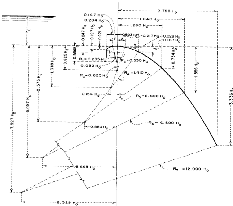
การออกแบบโค้งสันฝาย เมื่อ P \geq 0.5 H_0
